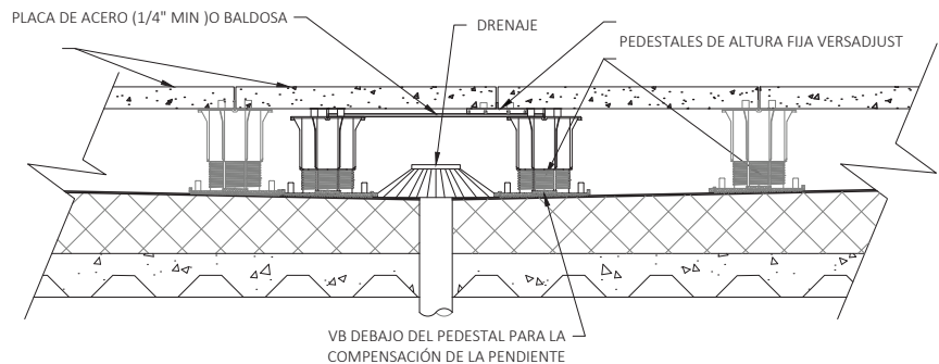
VISTA CORTE
